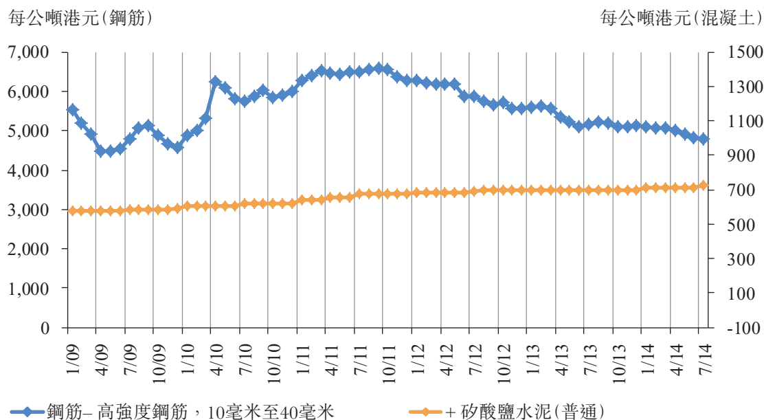
圖6：二零零九年至二零一三年香港鋼筋價格趨勢
